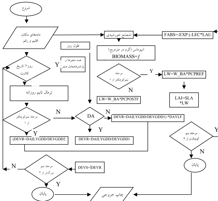
شکل ۱- الگوریتم مدل مورد استفاده برای شبیه‌سازی عملکرد. مرحله نمو ۱، گلدهی و مرحله نمو ۲ رسیدگی کامل را نشان می‌دهند. PCPREF و PCPOSTF ، DEVGDD ، DAILYGDD ، DAYLF ، DEVR ، SLA ، DEVS نشان می‌دهند. به ترتیب مرحله نمو، سطح ویژه برگ، سرعت نمو، طول روز، ترمال تایم روزانه، ترمال تایم مورد نیاز برای هر مرحله، ضریب تخصیص ماده خشک قبل از گلدهی و بعد از گلدهی را نشان می‌دهند.
