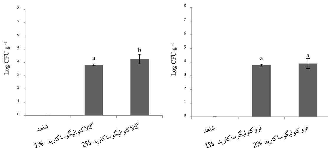
شکل ۲- اثر مقادیر مختلف پریبیوتیک‌های گالاکتوالیگوساکارید (الف) و فروکتوالیگوساکارید (ب) بر تعداد باکتری‌های اسیدلاکتیک (بر حسب لگاریتم واحد جدایه در گرم وزن روده) در میکروبیوتای روده‌ای بچه ماهی کلمه. ستون‌ها (SD± میانگین) با حروف متفاوت دارای اختلاف معنادار هستند ( P \text{ value} < 0.05 ).
