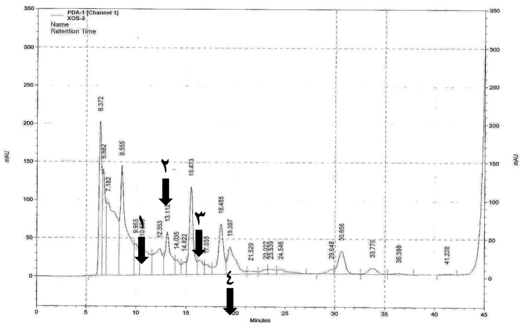
شکل ۴- منحنی کروماتوگراف بدست آمده برای تیمار سین بیوتیکی باکتری P. acidilactici با زایلوالیگوساکارید ۱، بوتریک اسید؛ ۲، لاکتیک اسید؛ ۳، پروپیونیک اسید؛ ۴، استیک اسید
