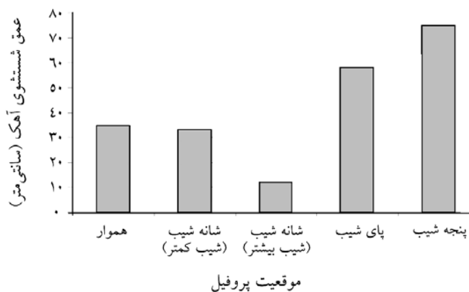
شکل ۲- عمق شستشوی آهک در موقعیت‌های مختلف شیب در منطقه گرگان.
