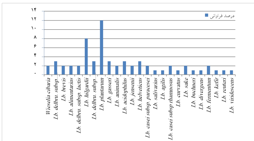
شکل ۲- پراکنده‌گی باکتری‌های میله‌ای شکل جدا شده از نمونه‌های چال.
