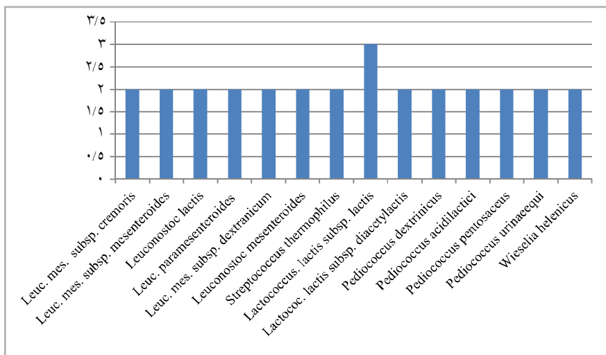
شکل ۱- پراکنده‌گی باکتری‌های غیرمیله‌ای شکل جدا شده از نمونه‌های چال.
